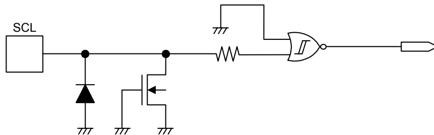
图22 SCL端子
