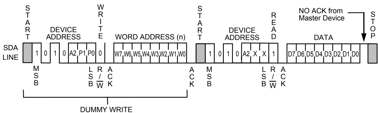
图20 随机读出
