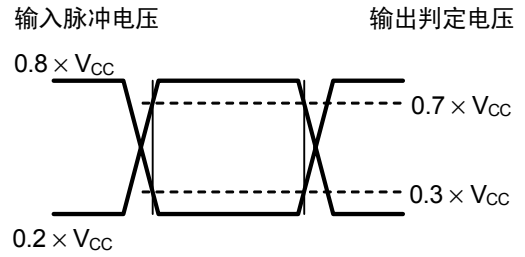
图7 AC测量输入、输出波形
