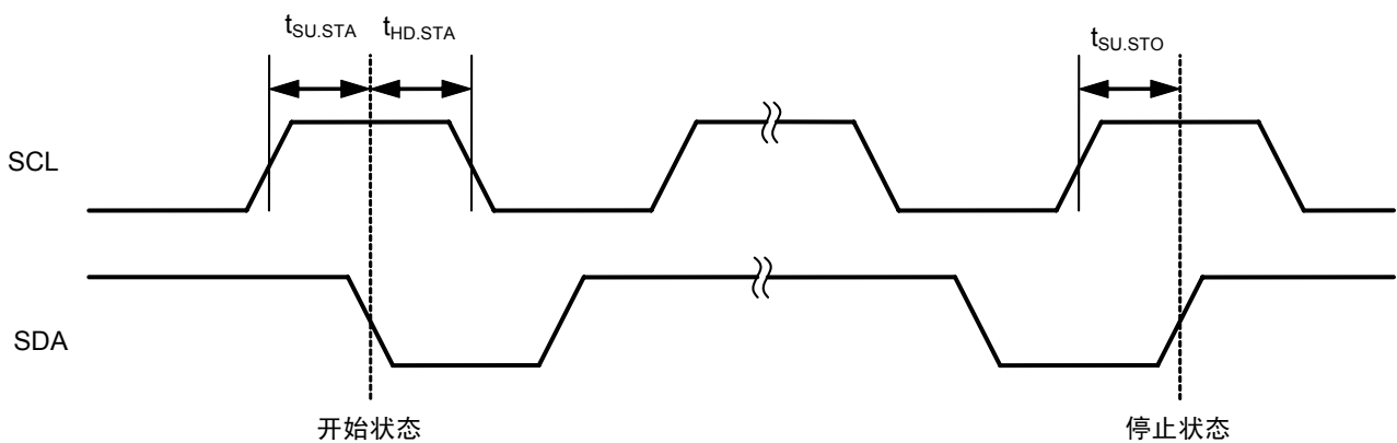
图11 开始 / 停止状态
