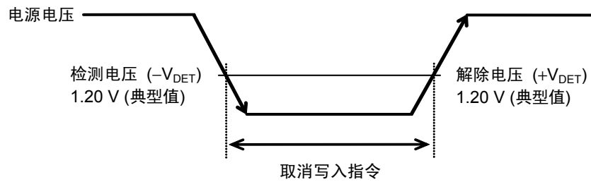
图22 低电源电压时的工作
