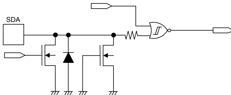
图24 SDA端子
