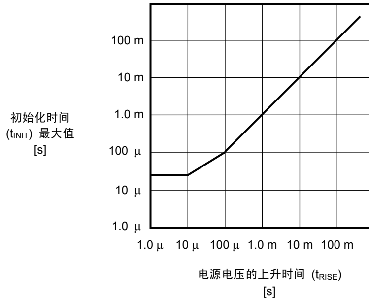
图30 S-24C08C的初始化时间
