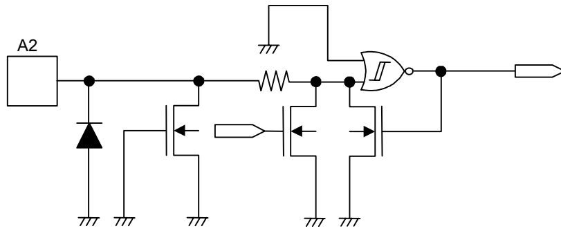
图26 A2端子
