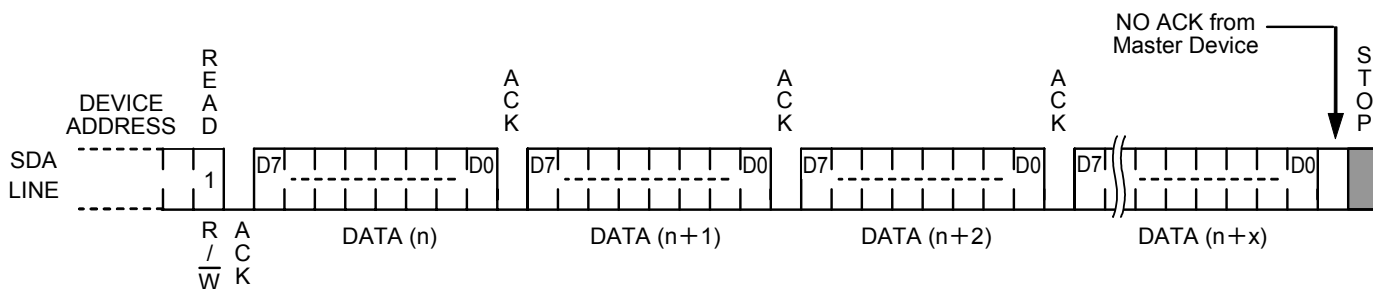
图21 顺序读出
