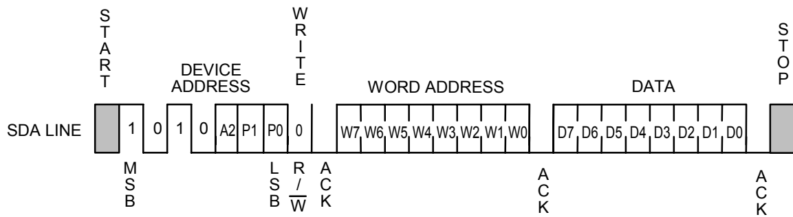
图15 字节写入
