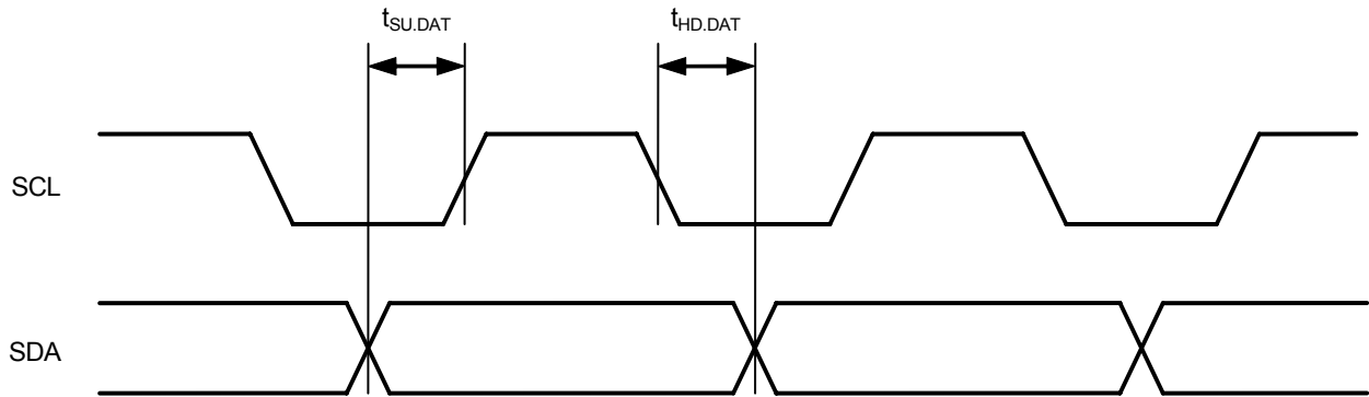
图12 数据传送定时
