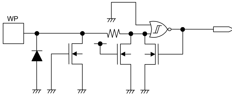
图25 WP端子
