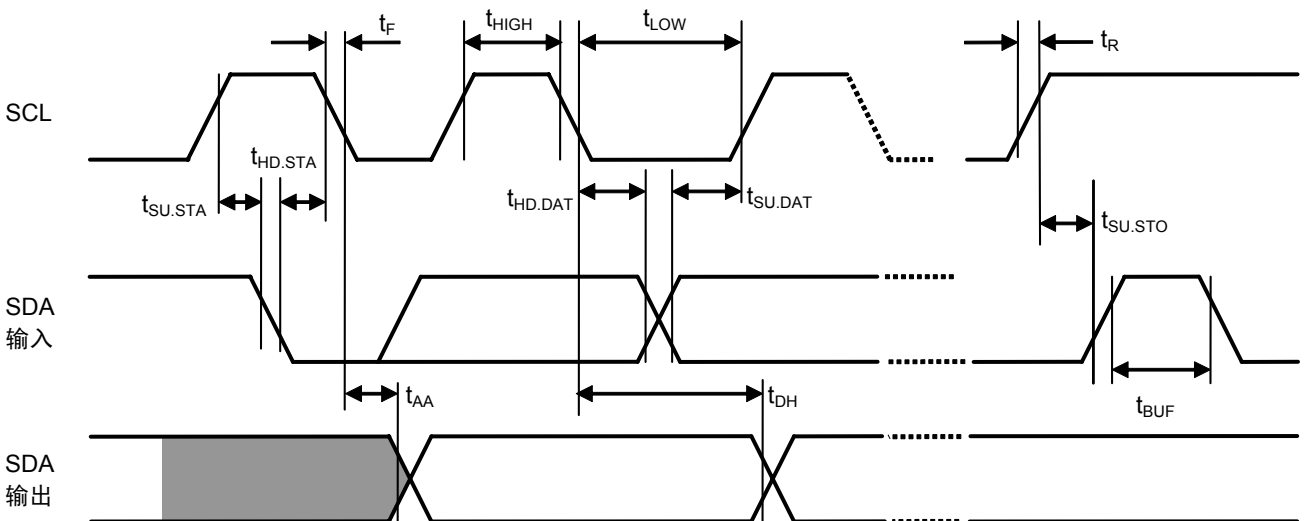
图8 总线定时
