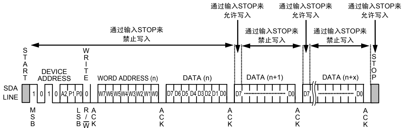
图33 通过在写入过程中输入停止状态来执行写入工作
