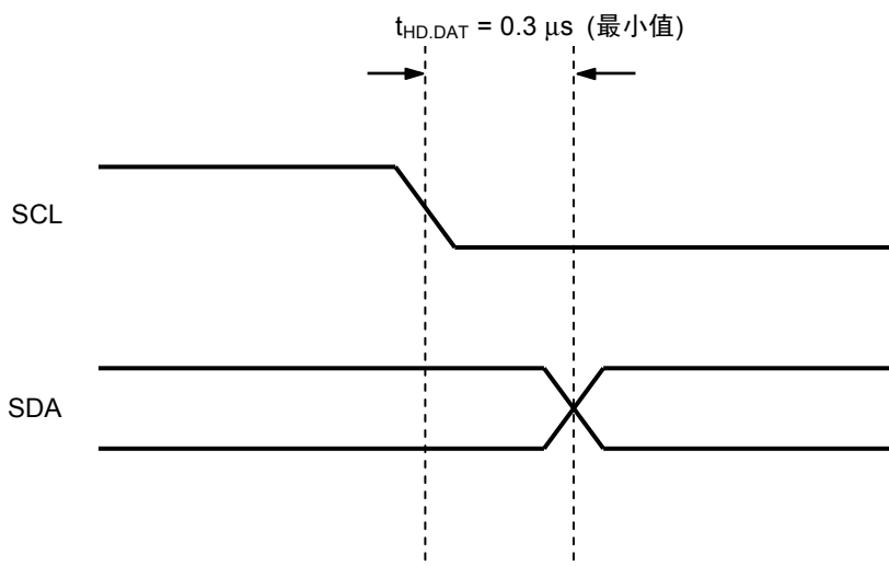
图31 S-24C08C的数据保持时间
