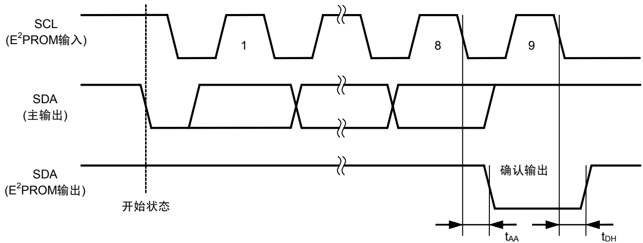
图13 确认输出定时
