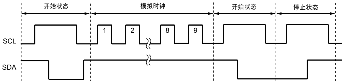
图27 S-24C08C的复位方法
