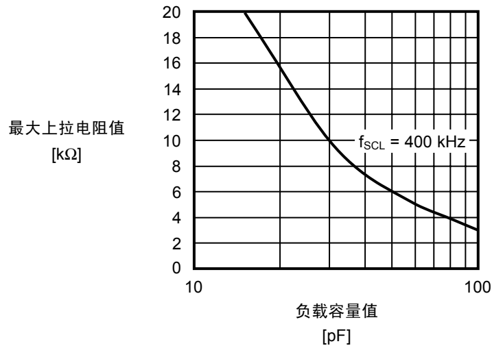
图10 输出负载
