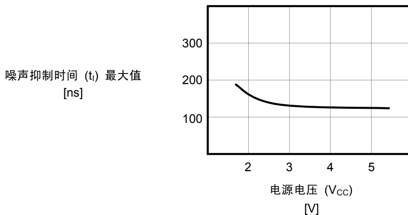
图32 SDA端子和SCL端子的噪声抑制时间
