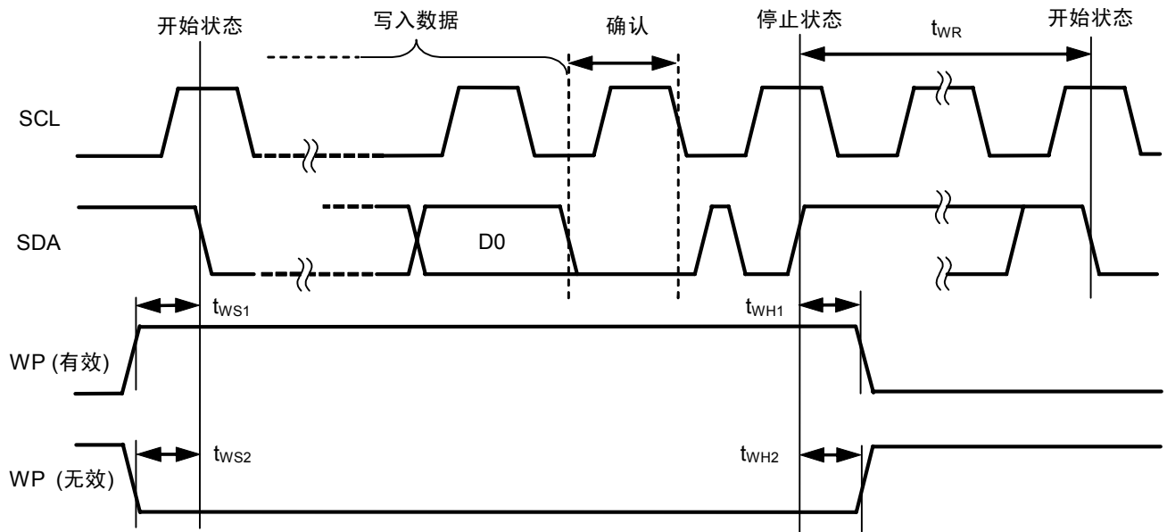
图9 写入周期定时
