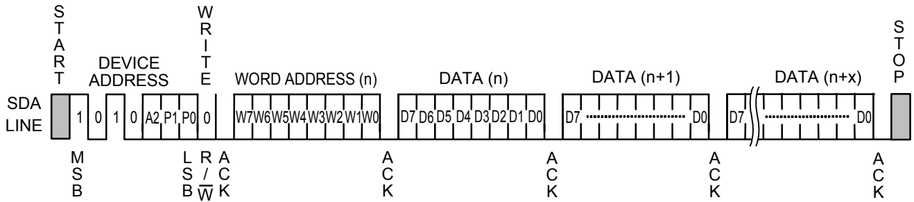
图16 页写入
