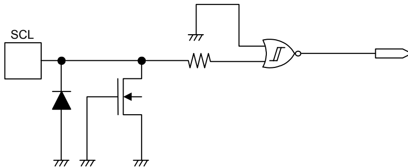
图23 SCL端子
