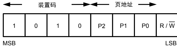
图14 装置地址
