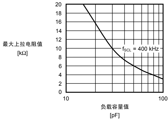
图10 输出负载
