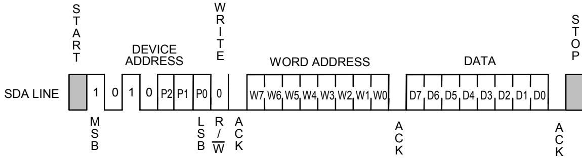
图15 字节写入
