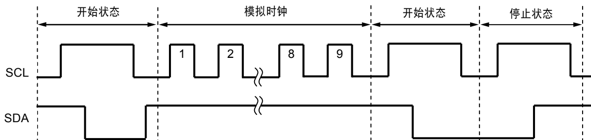
图26 S-24C16C的复位方法
