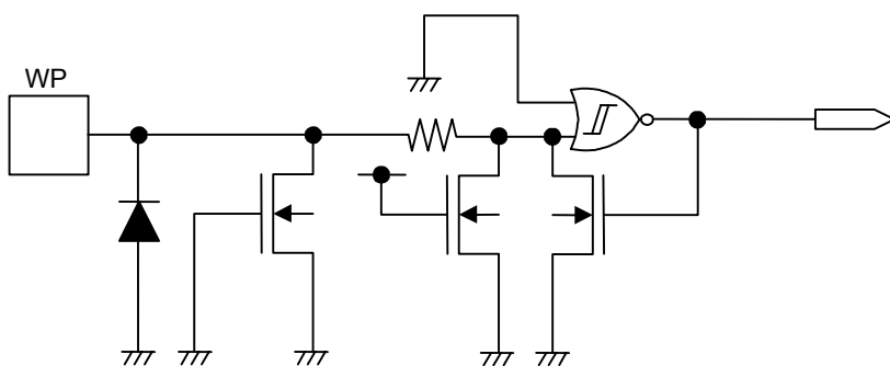
图25 WP端子
