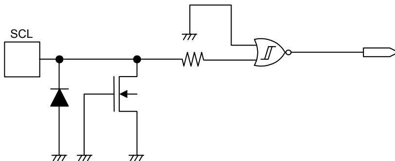
图23 SCL端子
