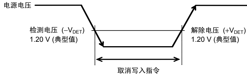
图22 低电源电压时的工作
