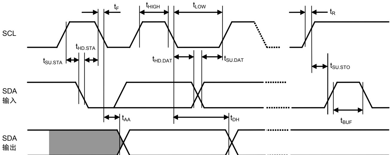
图8 总线定时
