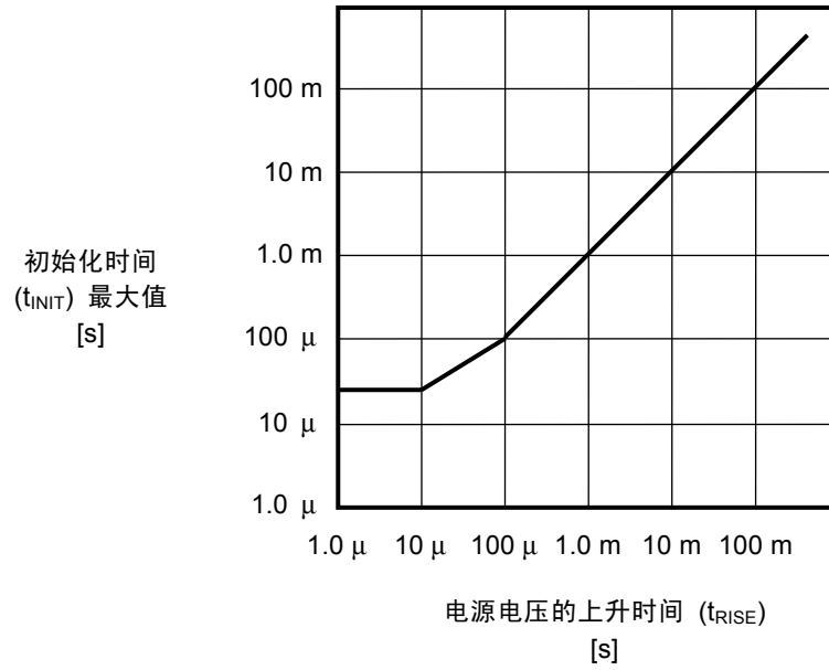
图29 S-24C16C的初始化时间
