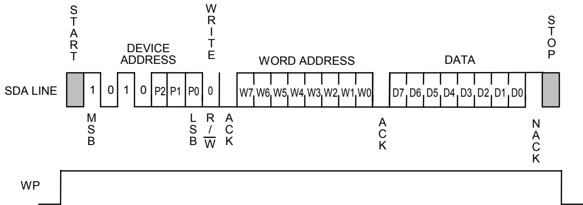
图17 写入保护
