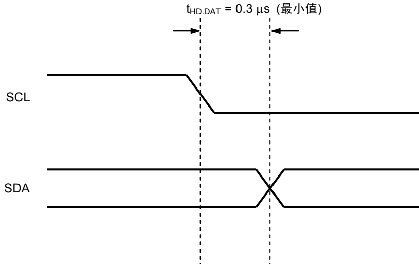
图30 S-24C16C的数据保持时间
