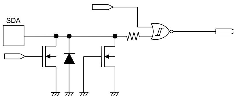
图24 SDA端子
