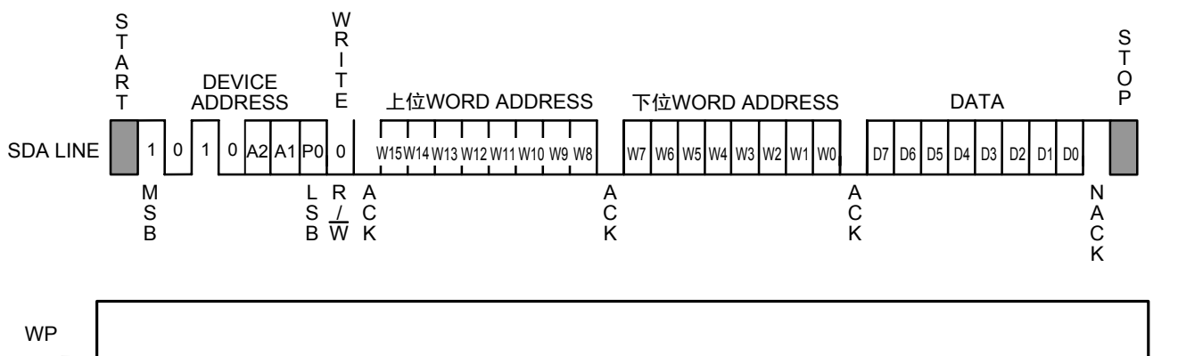
图13 写入保护
