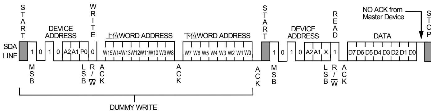
图16 随机读出
