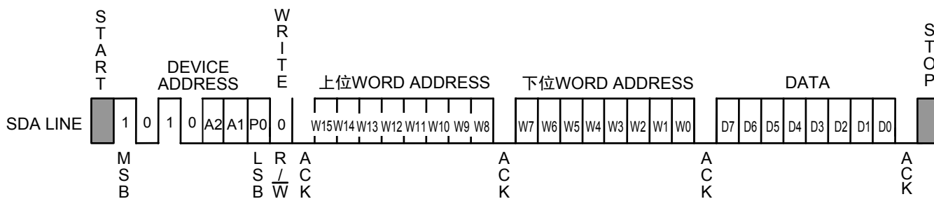
图11 字节写入
