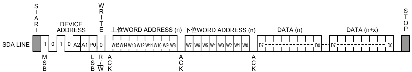
图12 页写入
