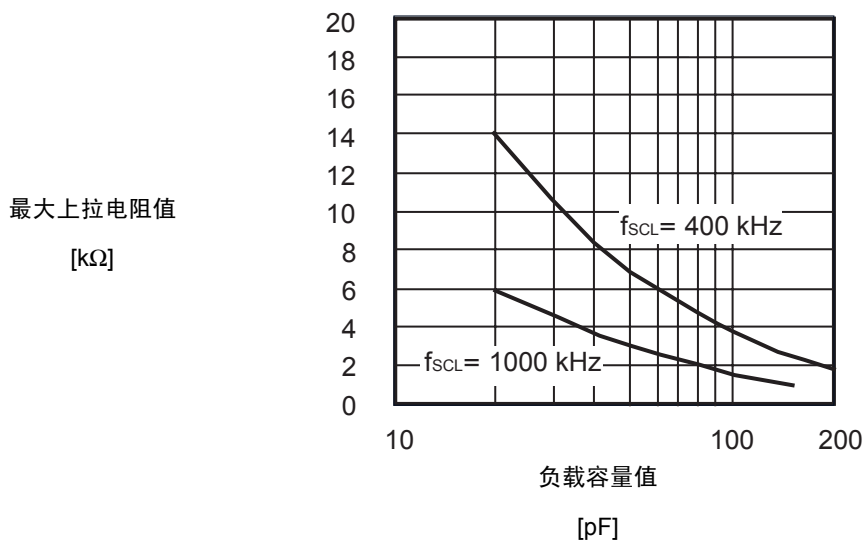
图6 输出负载
