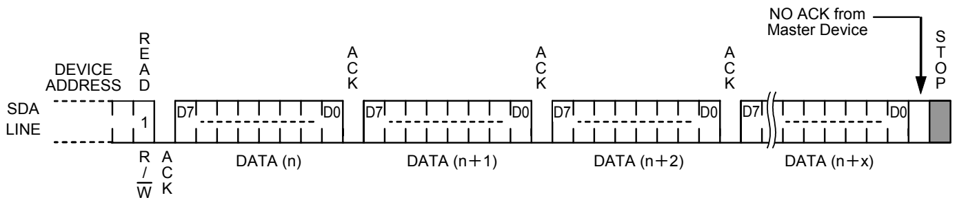
图17 顺序读出
