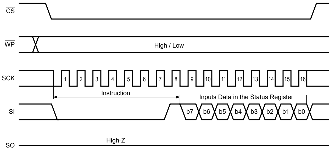
图17 WRSR 工作
