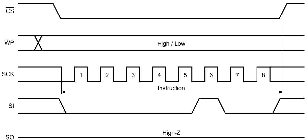
图15 WRDI工作
