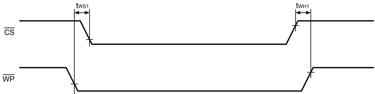
图10 保护写入有效定时
