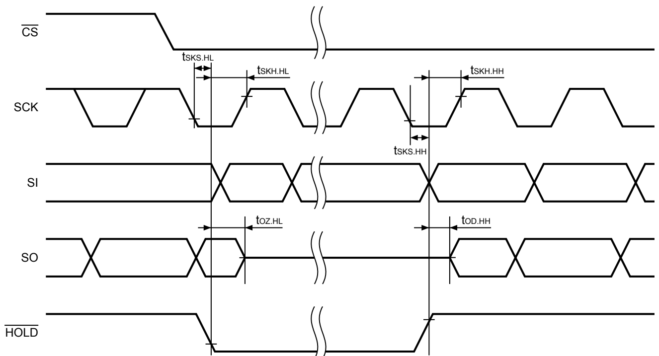
图7 保持定时
