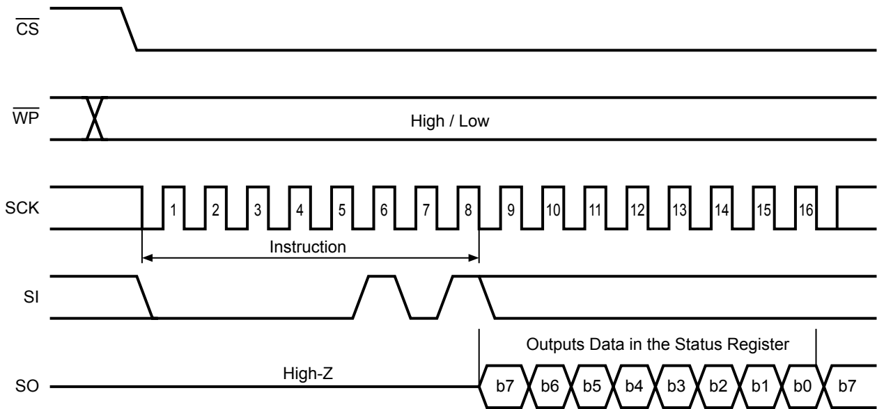
图15 RDSR 工作
