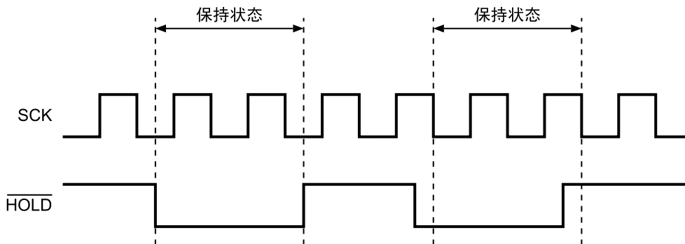
图20 保持工作
