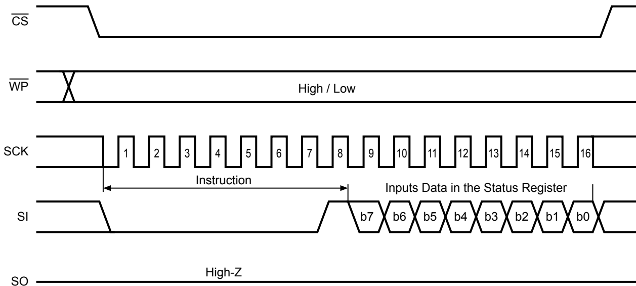
图16 WRSR 工作
