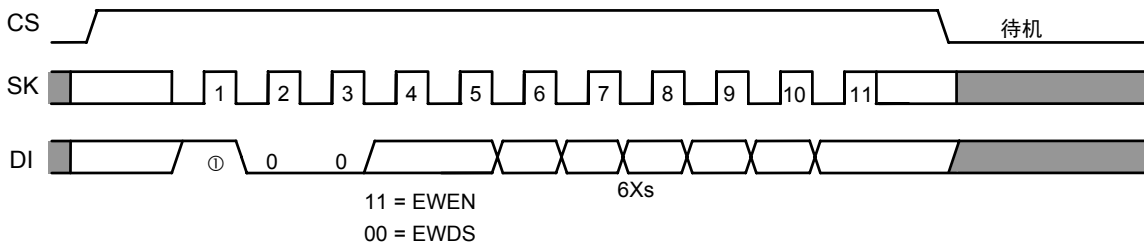
图19 允许或禁止写入定时 (S-93C56B、S-93C66B)
