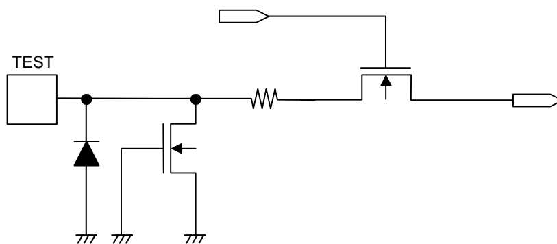
图25 TEST端子
