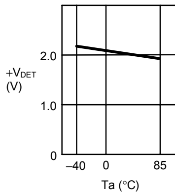
1.32 低电源解除电压 +V_{DET} —周围温度 T_a
