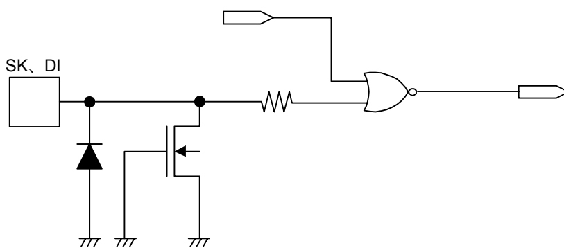
图15 SK、DI端子
