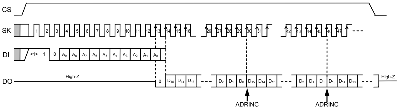
图5 读出定时
