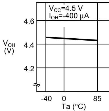
1.17 高电位输出电压 V_{OH} —周围温度 T_a
