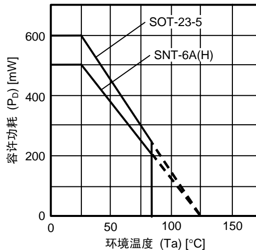
图5 封装容许功耗
