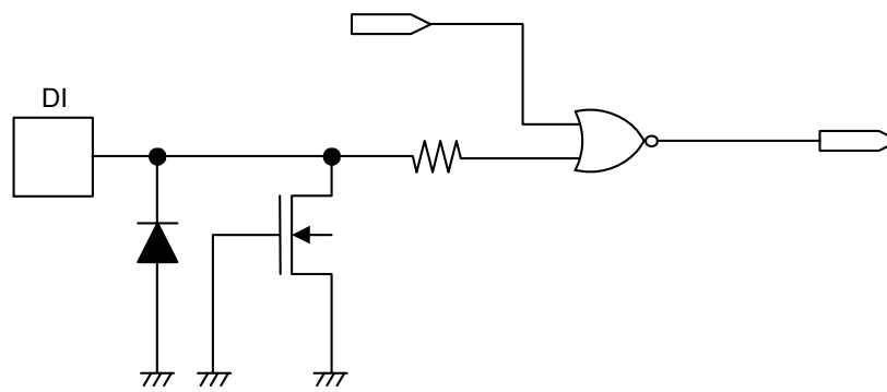
Figure 23 DI Pin
