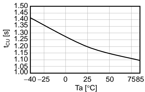
(5) t_{CU}-T_a
