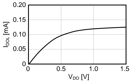
(4) I_{DOL} - V_{DO}
