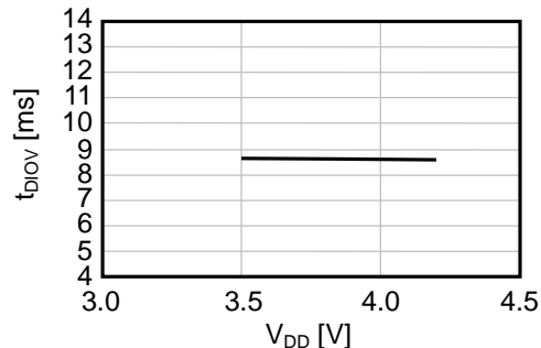
(8) t_{DIOV}-V_{DD}
