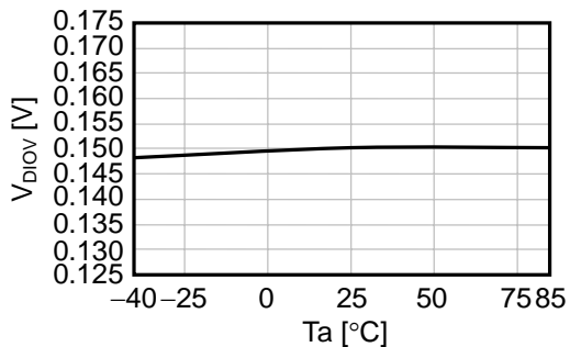
(7) V_{DIOV}-T_a
