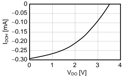
(3) I_{DOH} - V_{DO}
