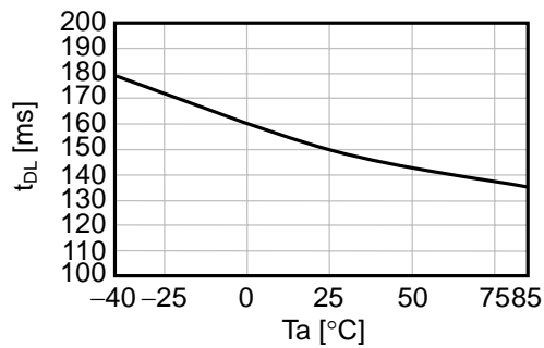
(6) t_{DL}-T_a
