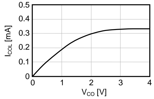
(2) I_{COL} - V_{CO}
