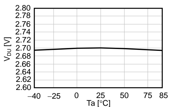
2.3 V_{DU}-T_a
