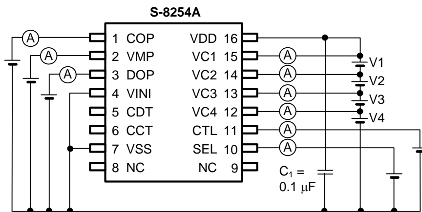
図8 測定回路5
