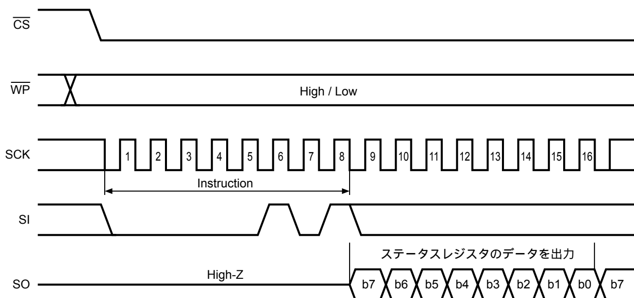
図 14 RDSR 動作
