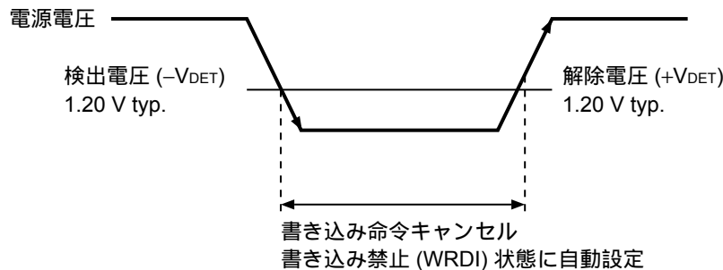
図 21 低電源電圧時の動作 (S-25A640B)
