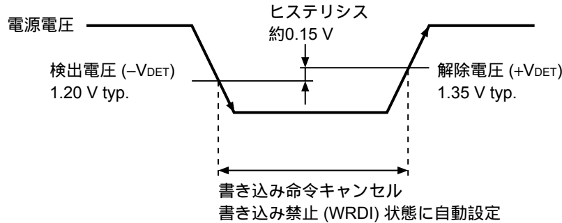
図 20 低電源電圧時の動作 (S-25A640A)
