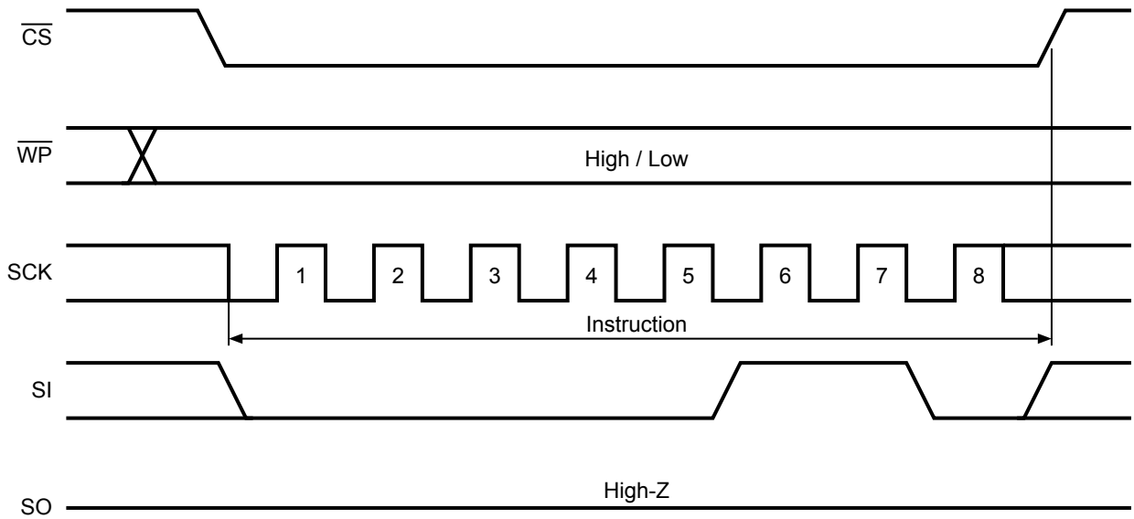
図 12 WREN 動作
