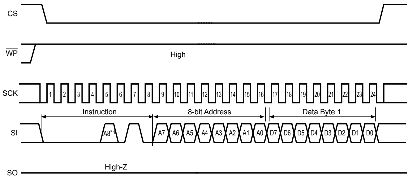
図 17 WRITE 動作 (1 バイト) (S-25C010A/020A)
