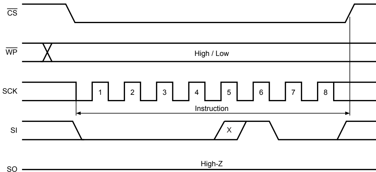
図 12 WRDI 動作
