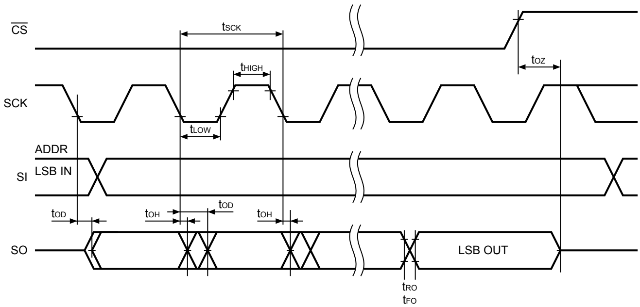
図 6 シリアル出カタイミング
