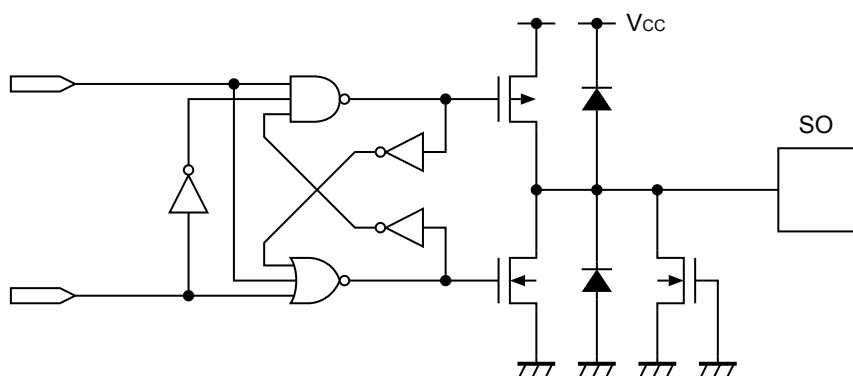
図 25 SO 端子
