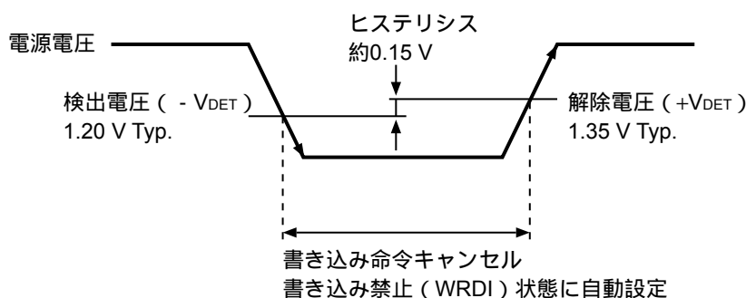
図 22 低電源電圧時の動作
