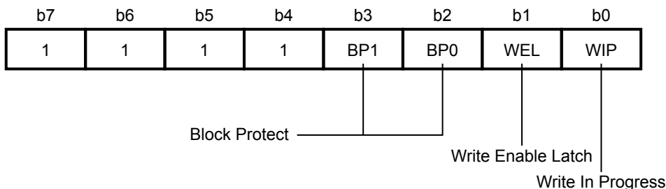
図9 ステータスレジスタ構成図
