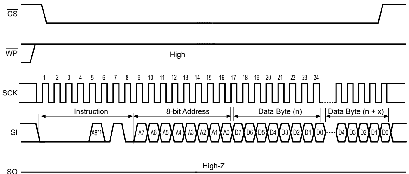
図 19 WRITE 動作 (ページ) (S-25C010A/020A)
