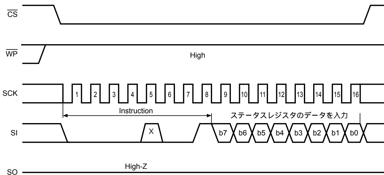
図 14 WRSR 動作
