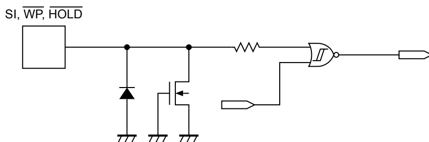
図 21 SI, \overline{WP} , \overline{HOLD} 端子
