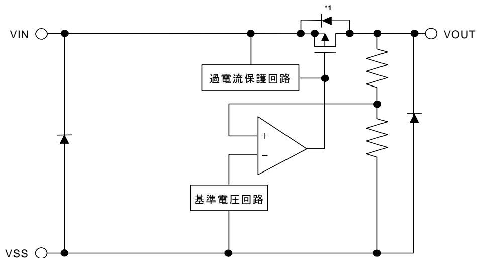
(1) パワーオフ機能なし(パッケージ : SOT-89-3)
