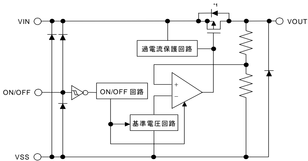
(2) パワーオフ機能あり(パッケージ : SOT-89-5、6-Pin HSON(A))
